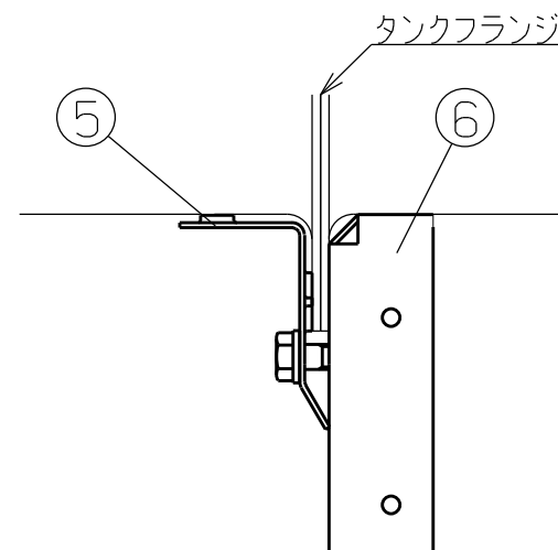
ホームタンクへの取り付け部詳細
