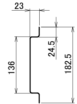
断面図(共通)
