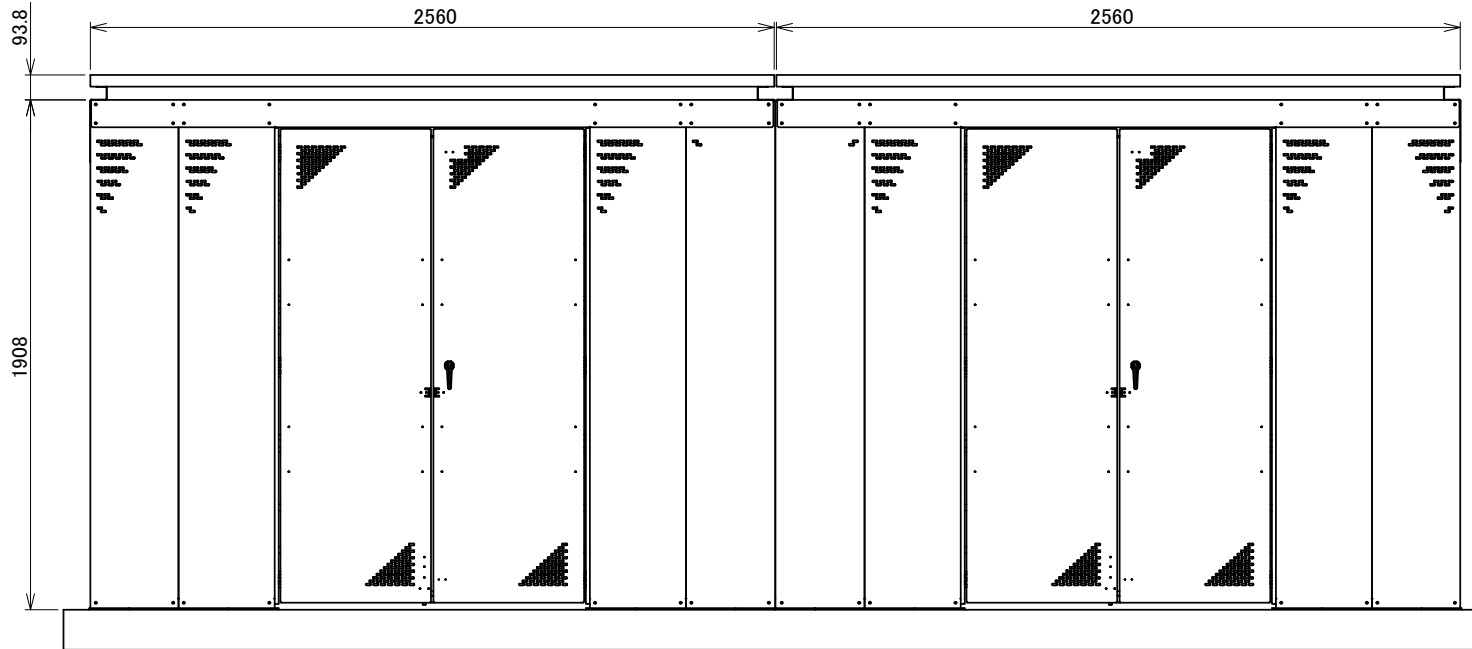
承認図
