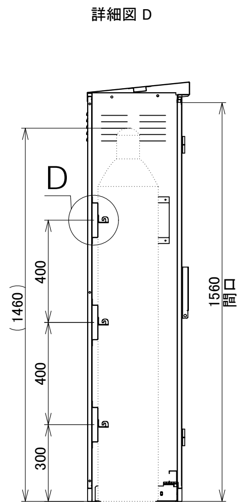
断面図 A-A
