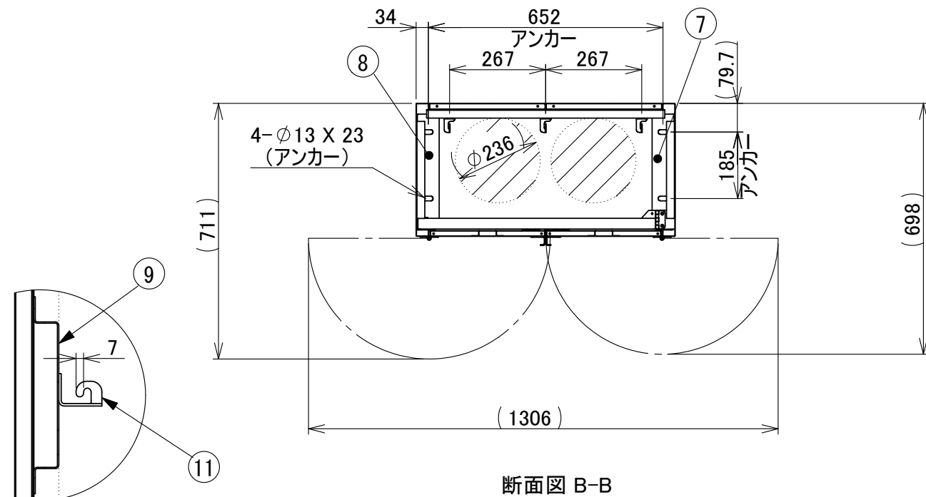
詳細図 D
