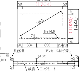
基礎伏図
