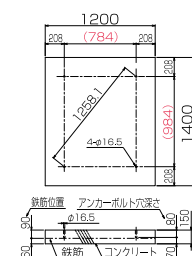
基礎伏図
