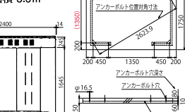
背面図
