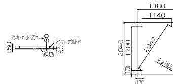
基礎伏図
