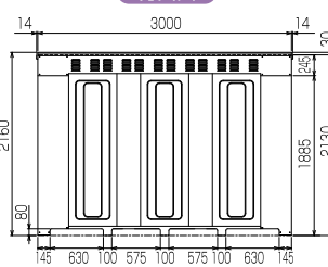
背面図
