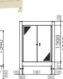
正面図
