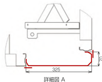
詳細図 A
