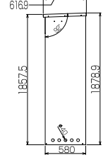
側面図
