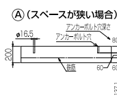
基礎伏図
