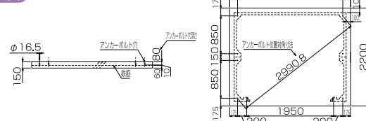
基礎伏図
