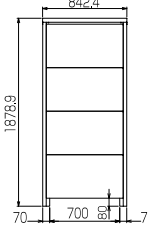
背面図
