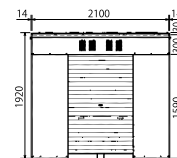
正面図
