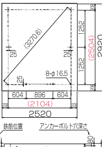
基礎伏図
