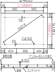
基礎伏図
