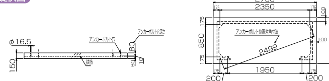
基礎伏図
