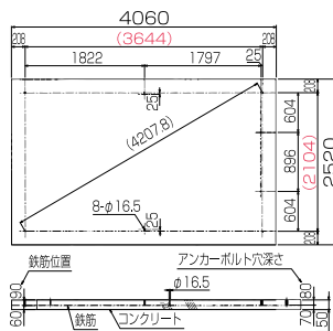
基礎伏図
