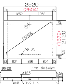
基礎伏図
