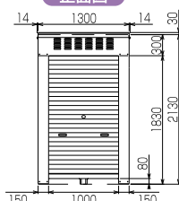
正面図
