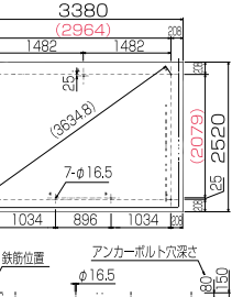
基礎伏図
