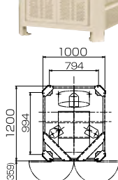
平面図
