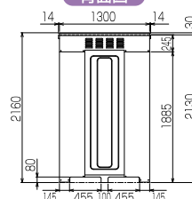
背面図
