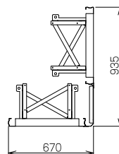
平面図 (取り付け向きを90° 変えた場合)
