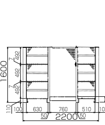
正面図
