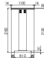
背面図
