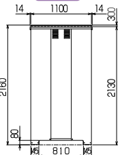
背面図
