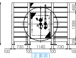
正面図
