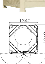
平面図
