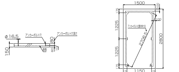
正面図
