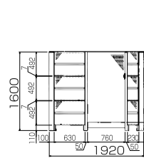
正面図
