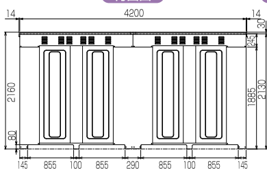
背面図
