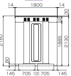
背面図
