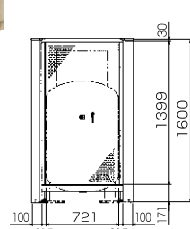
正面図
