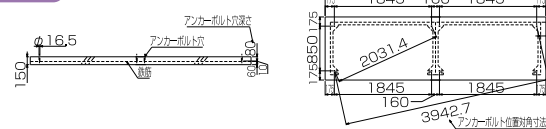
基礎伏図
