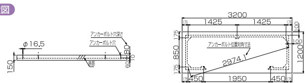
正面図
