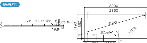
基礎伏図
