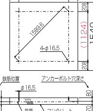
基礎伏図
