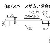
背面図
