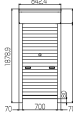
正面図
