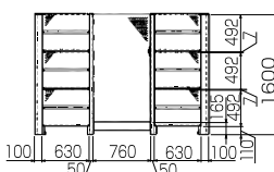
正面図
