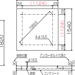
基礎伏図
