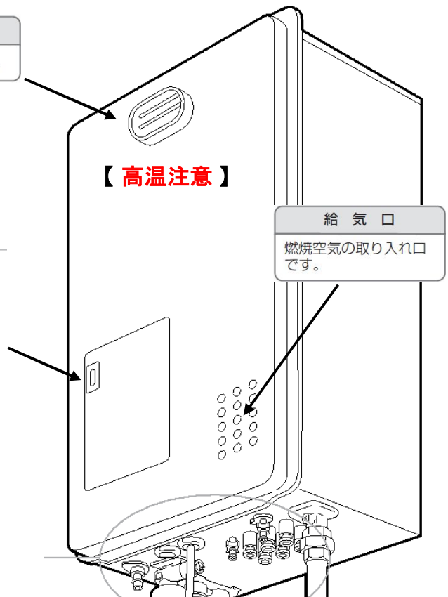
ボイラー本体の各部名称
