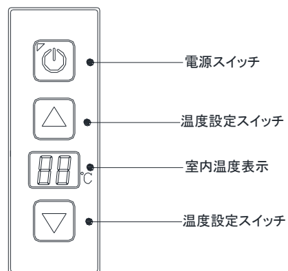
《操作パネル詳細図》
