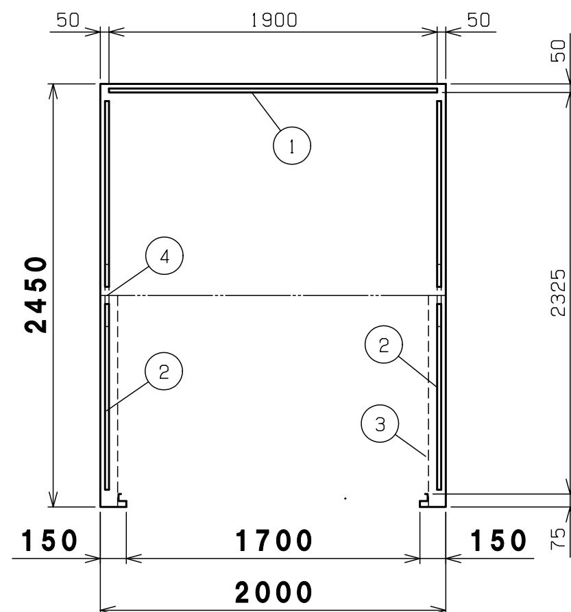
内面図
