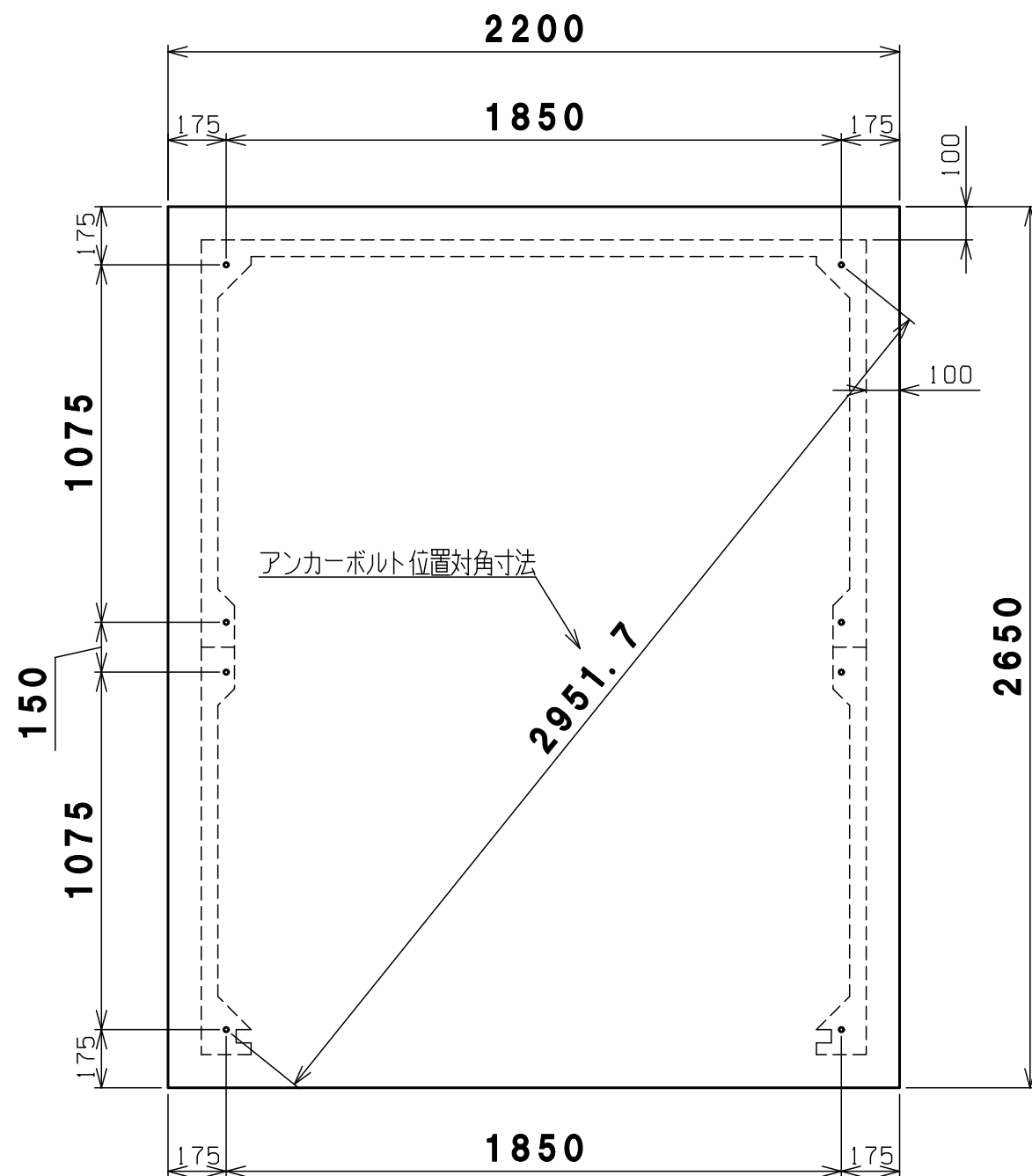
基礎平面図
