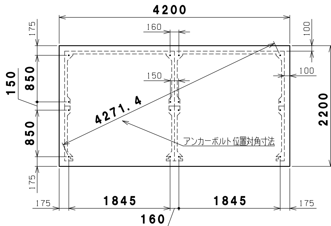
基礎平面図
