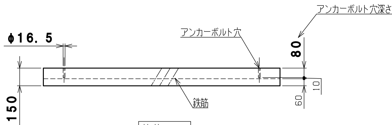
基礎正面図
