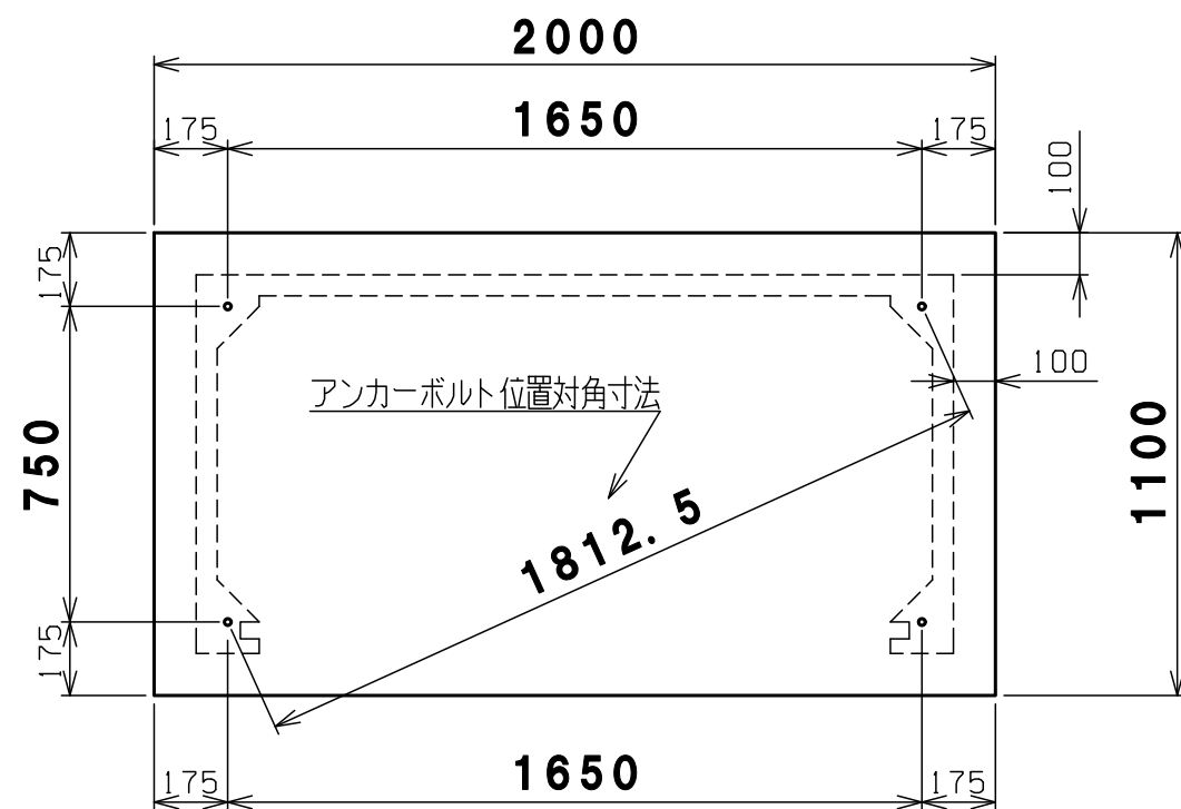
基礎平面図
