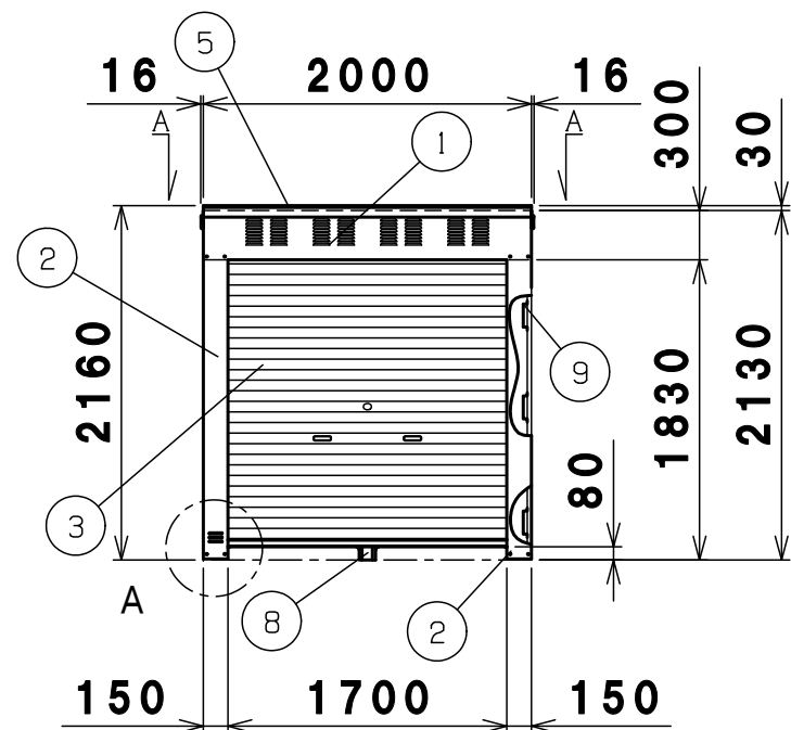
正面図
