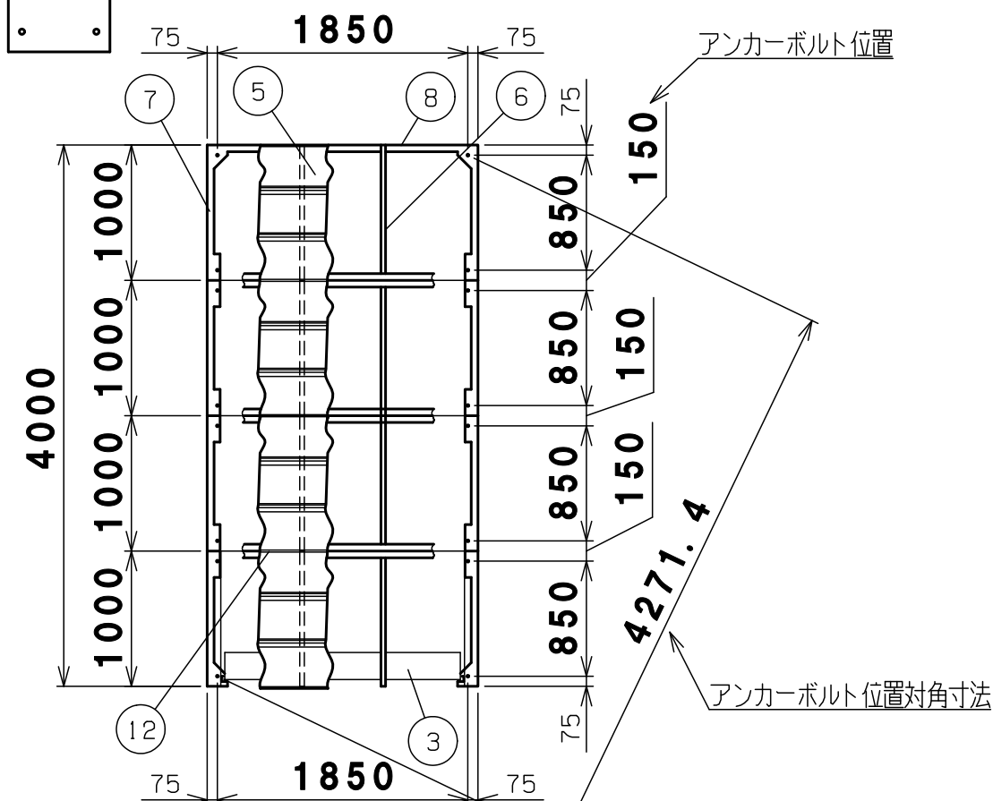
平面図-A-A
