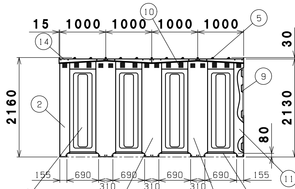
側面図
