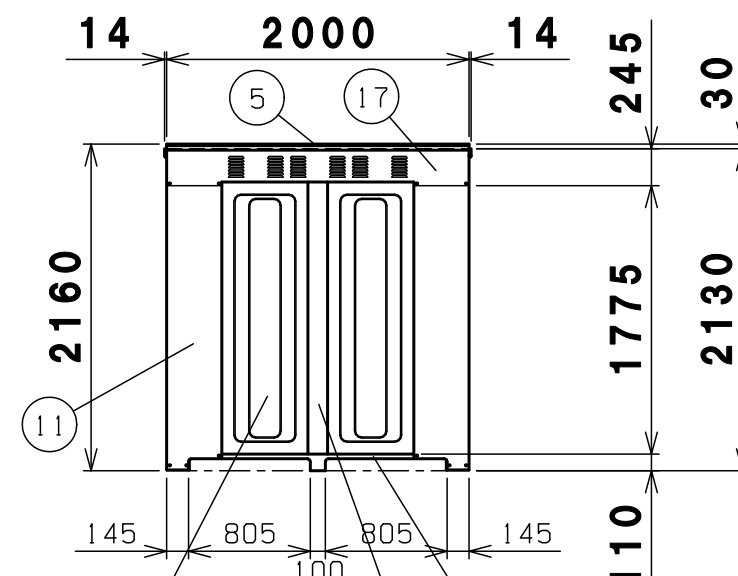
背面図
