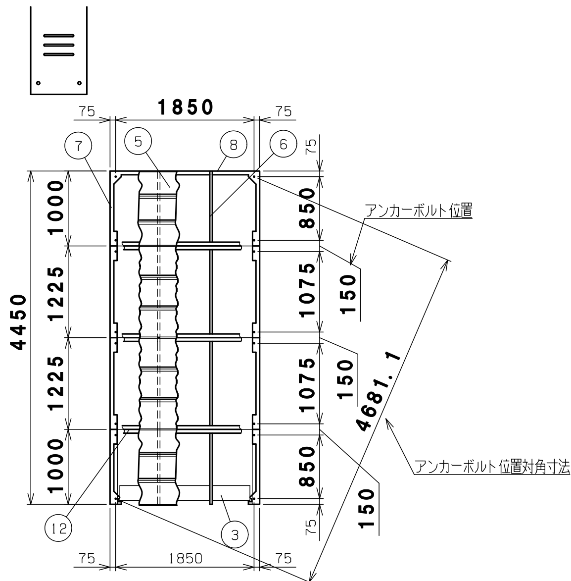
平面図-A-A
