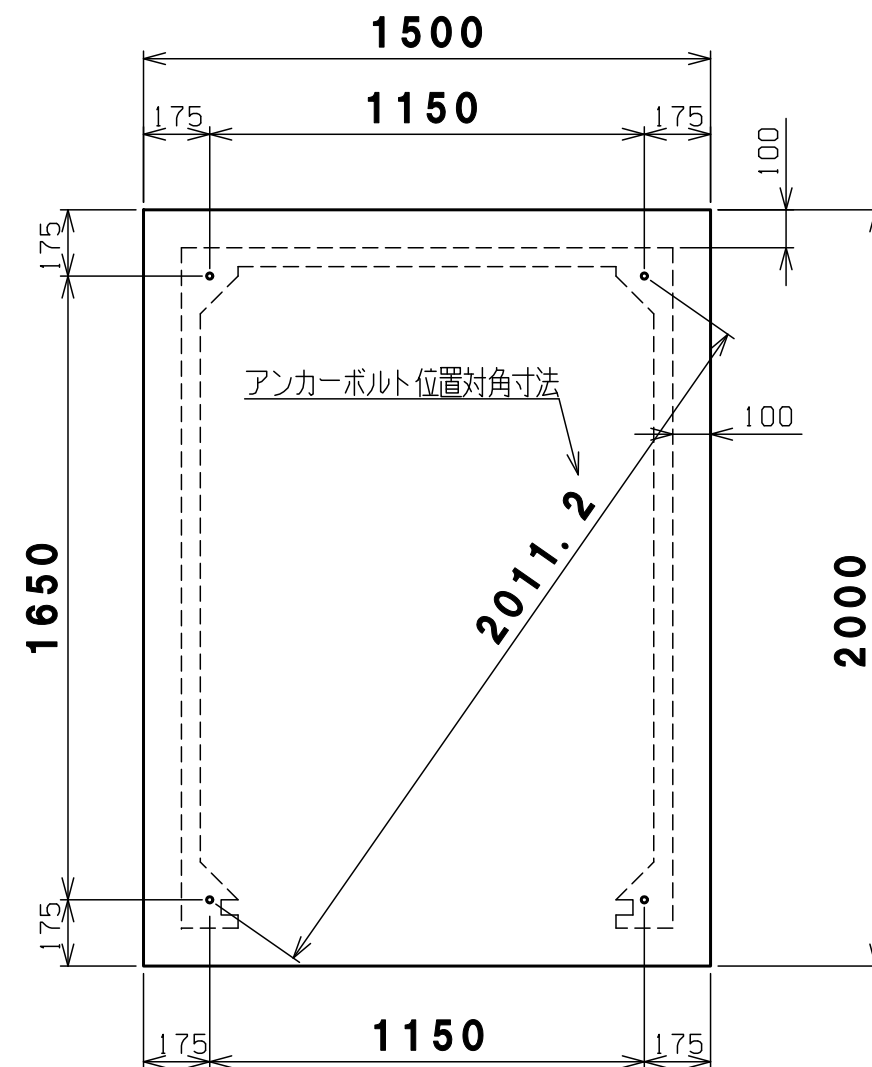
基礎平面図
