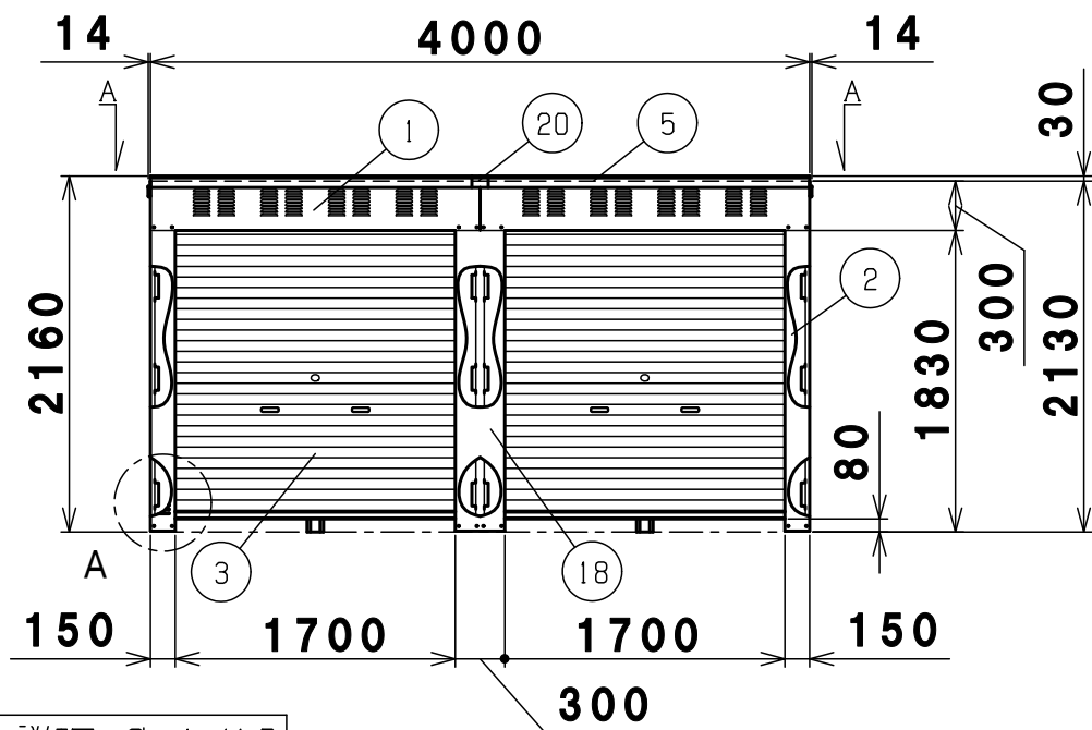
正面図
