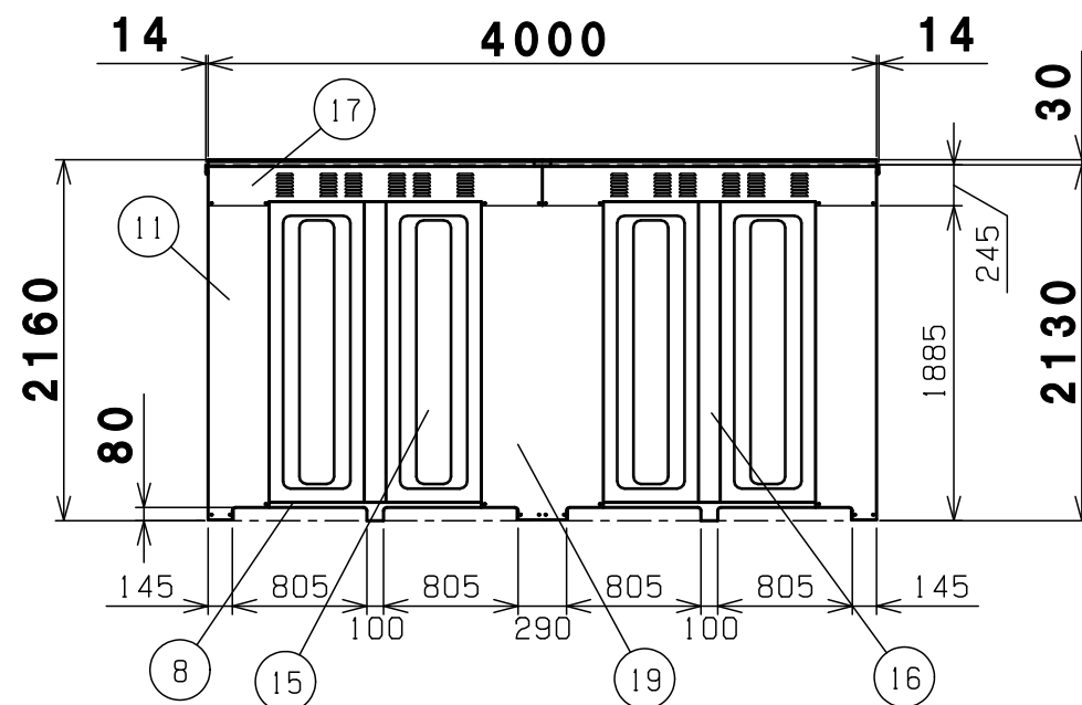
背面図
