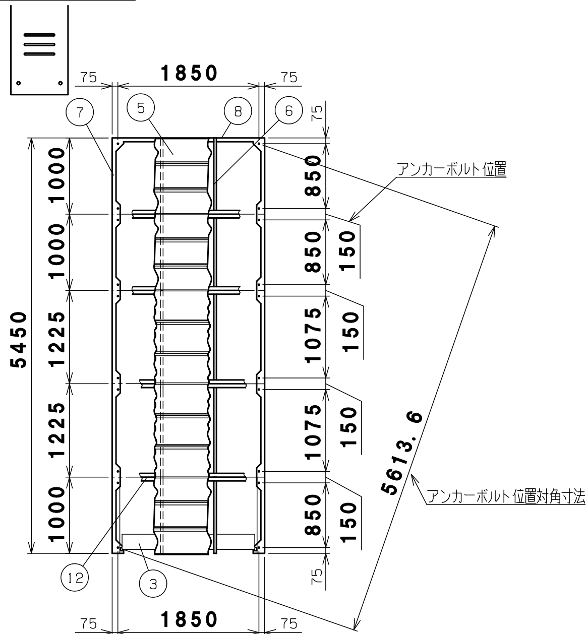
平面図-A-A
