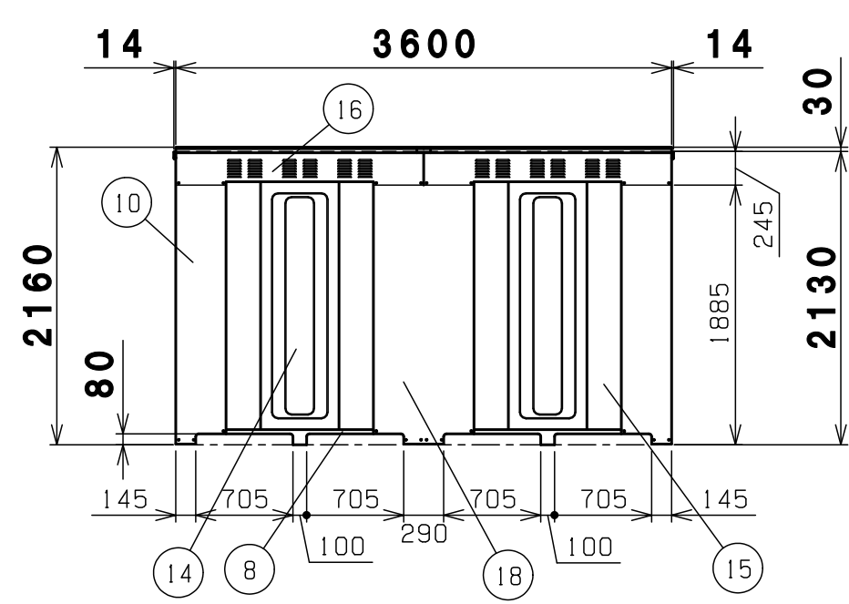
背面図
