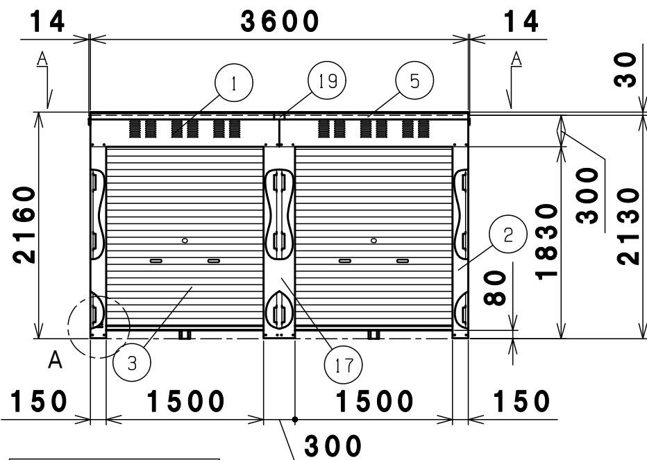
A-詳細図 S=1/10
