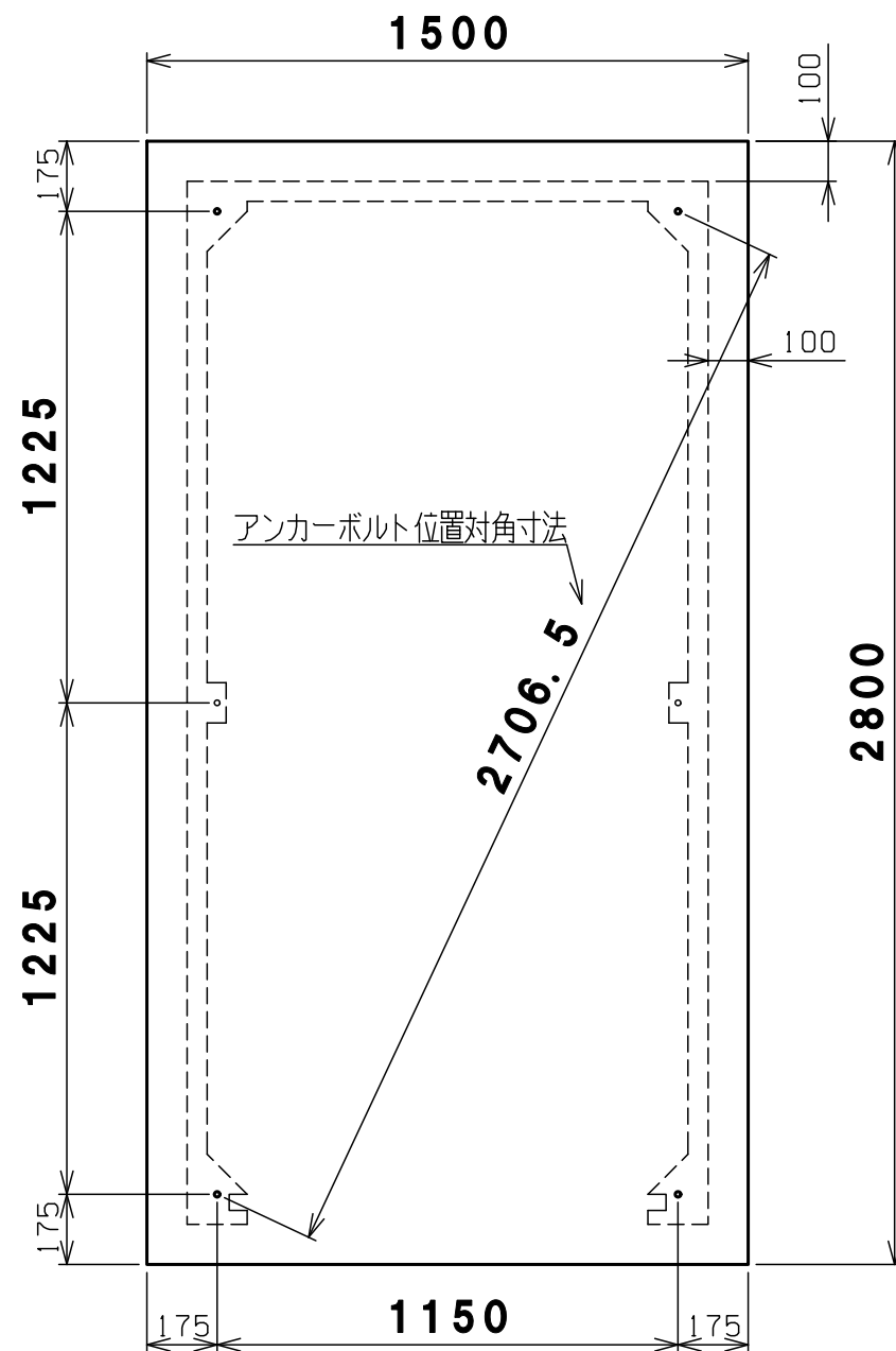
基礎平面図
