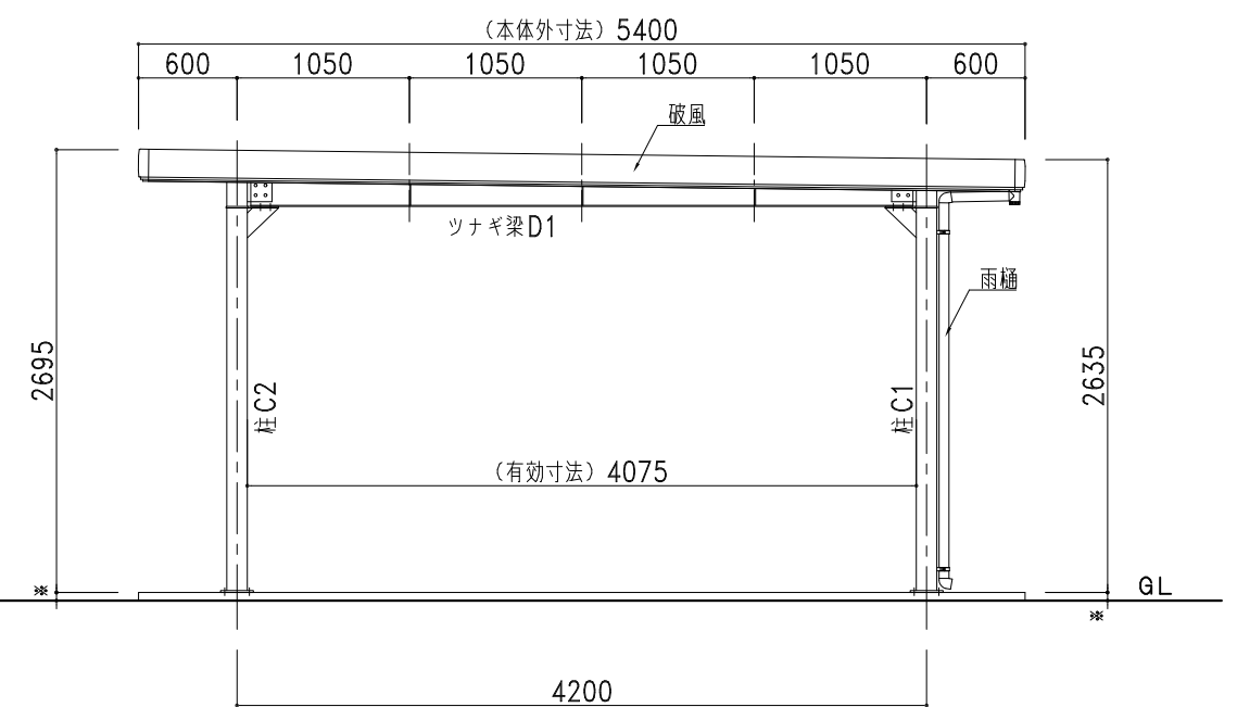
側面図
