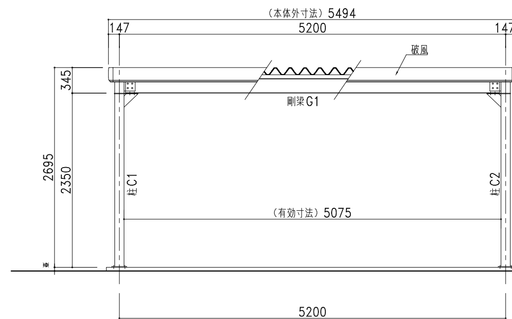
正面図
