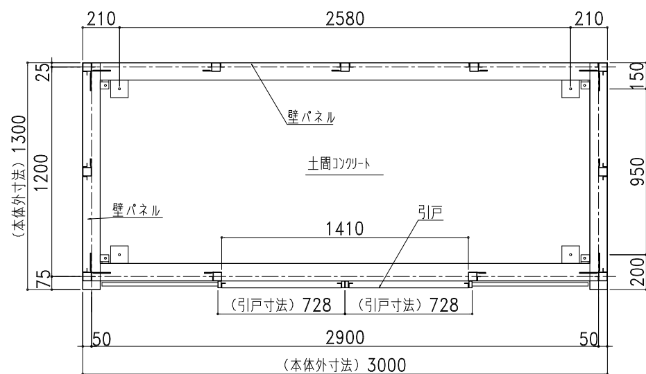
平面图
