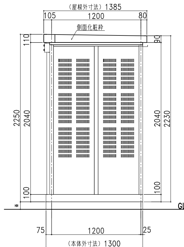
側面図
