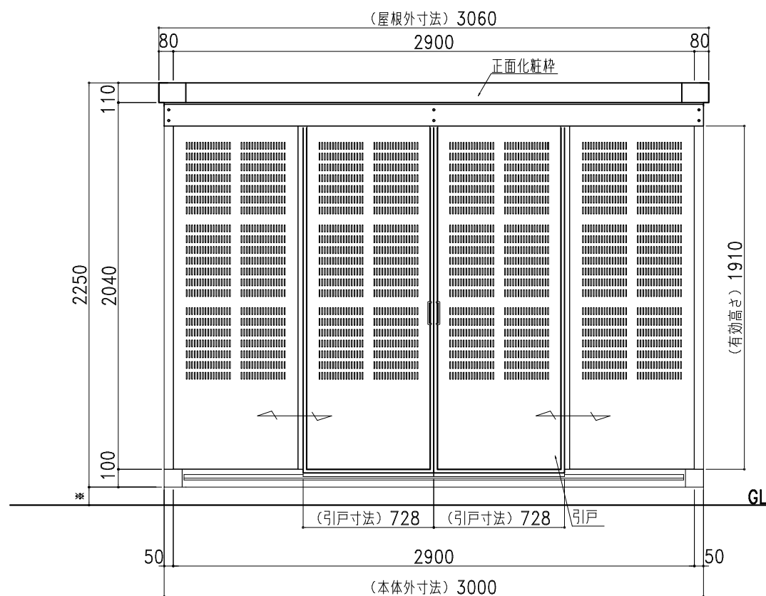
正面义
