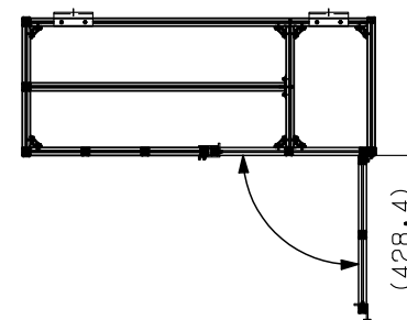
A-A断面図
