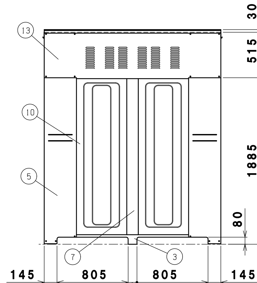
背面図
