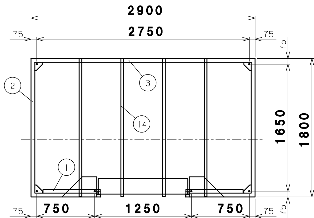
平面図 A-A
