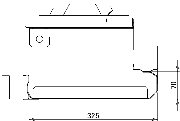
詳細図 A
