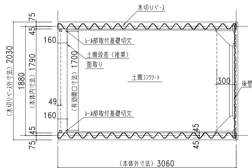
平面图
