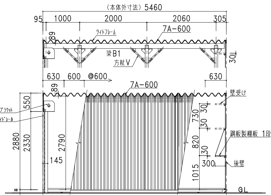
側面図・断面図
