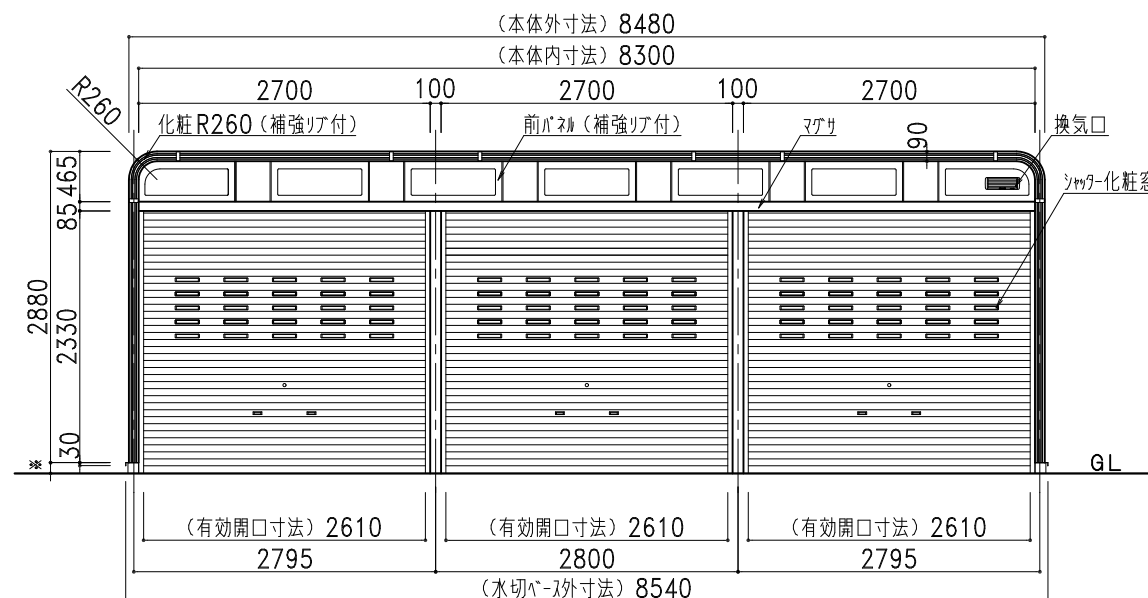
正面図
