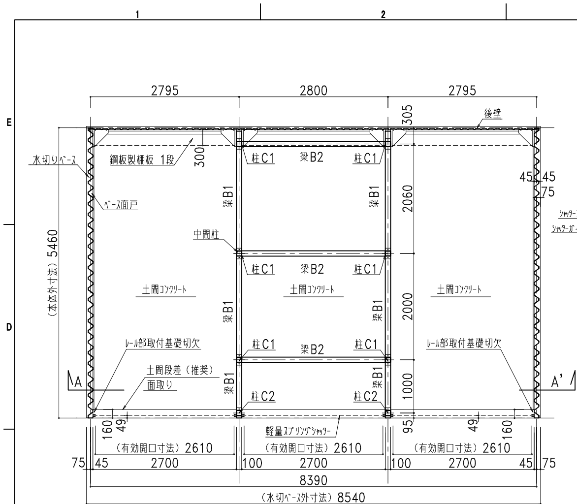
平面图
