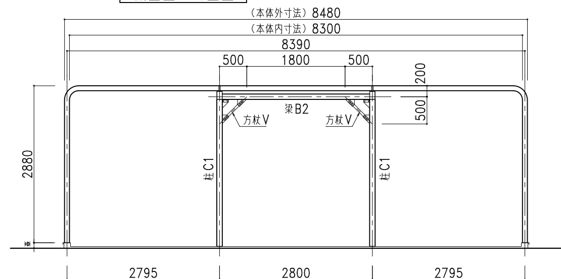
A-A' 断面图
