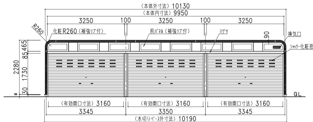
正面図
