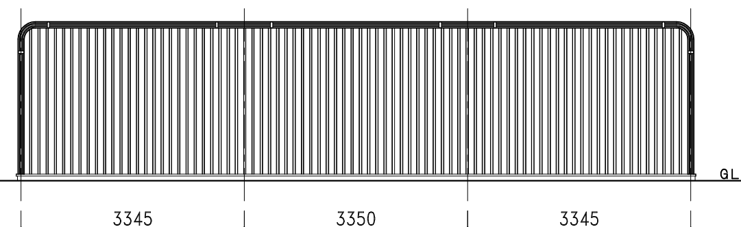
側面図・断面図
