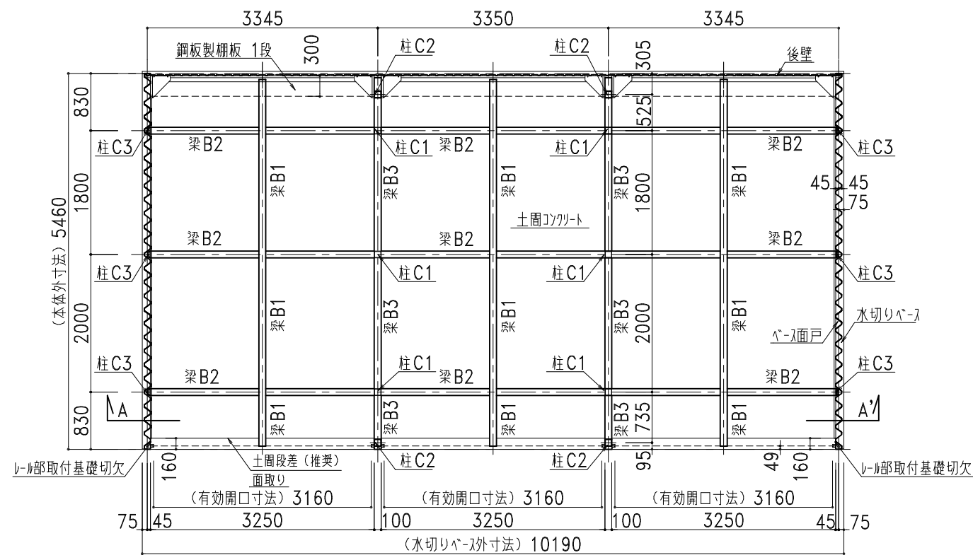
平面図
