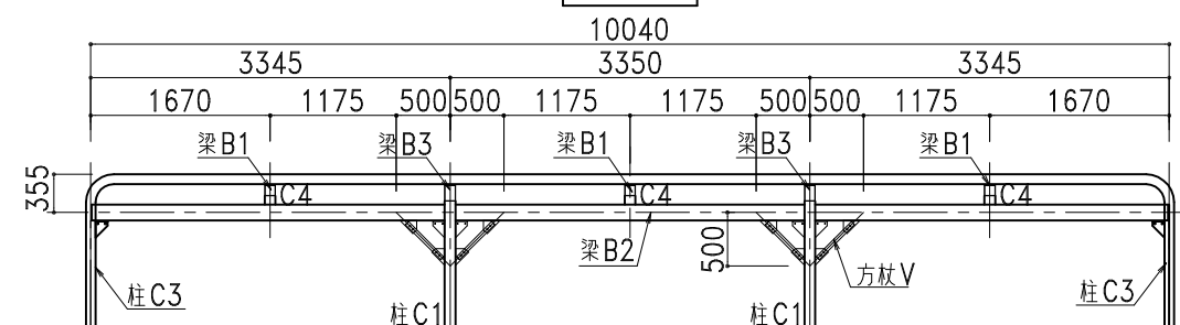
A-A' 断面图
