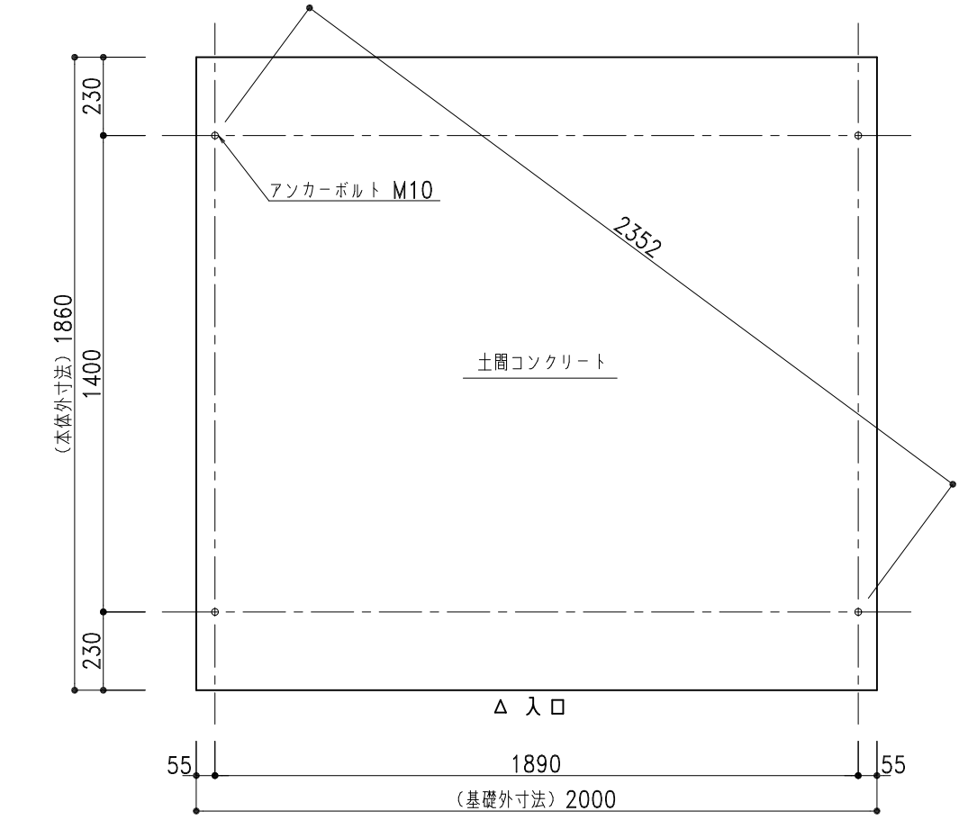
基礎伏図 1/20
