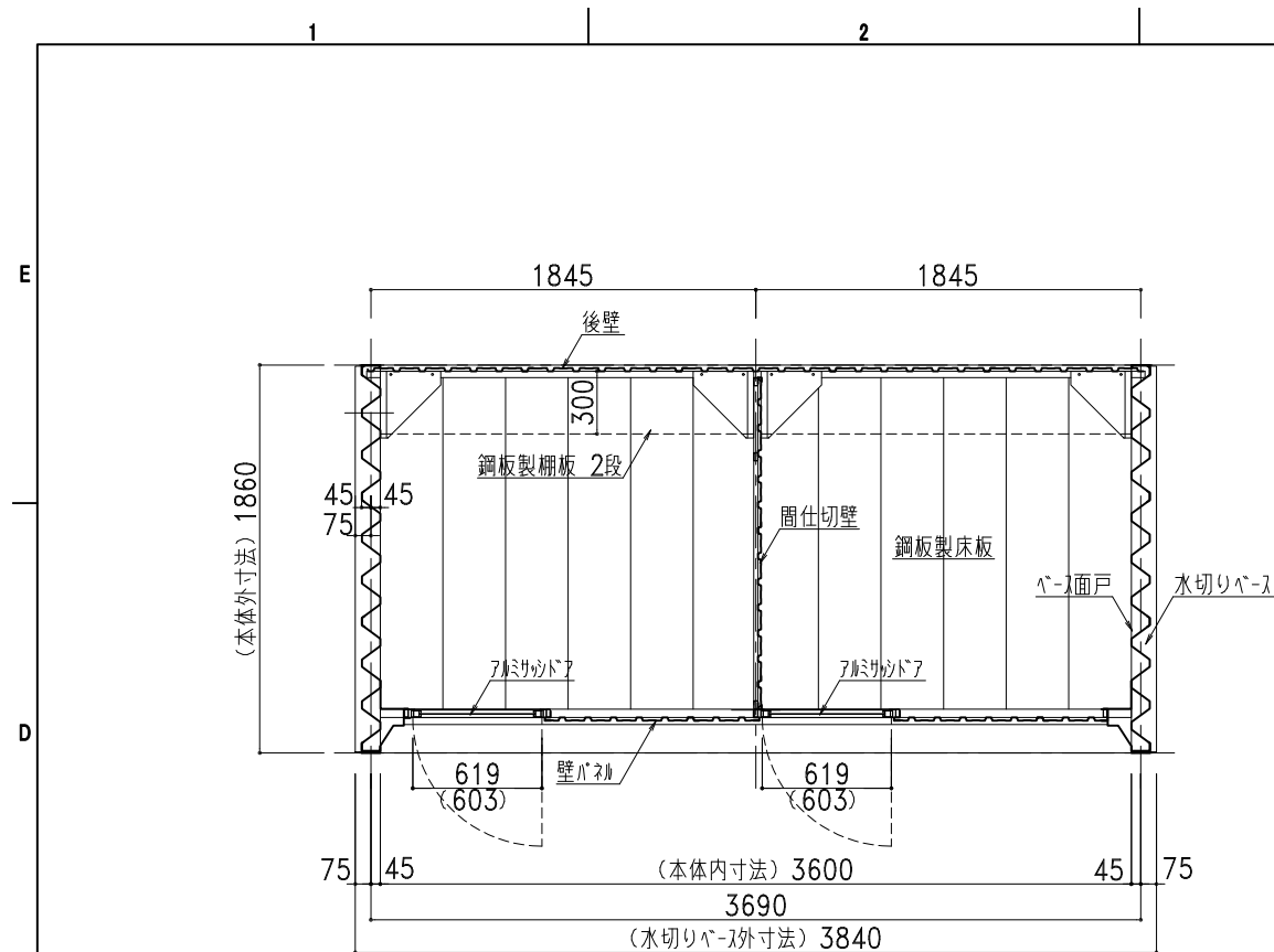
平面图
