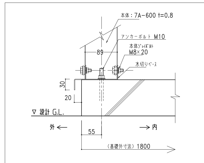
へ-λ取付図 1/5
