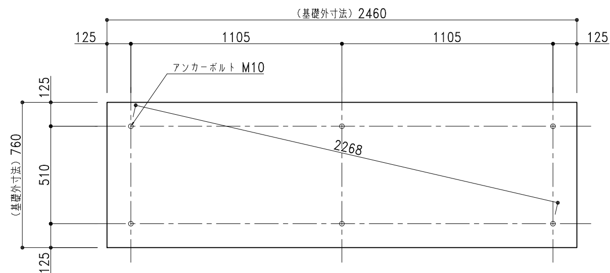
基礎伏図 1/20
